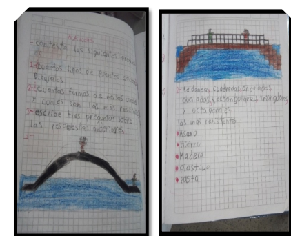
Figura 4. Respuestas Estudiantes 402
